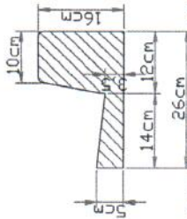
DETALHE DO MEIO-FIO SEM ESCALA
