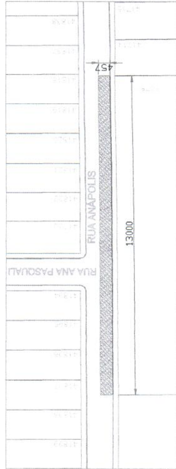
PLANTA BAIXA RUA ANÁPOLIS SEM ESCALA
